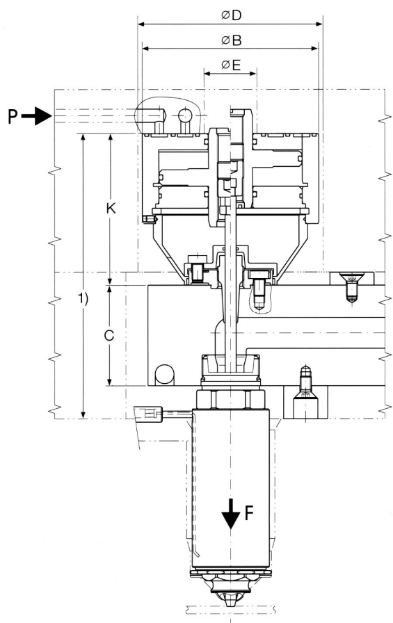
DFQ — ネジ込み式
